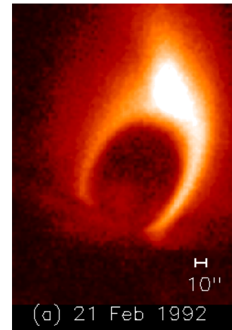
Solar Flare
